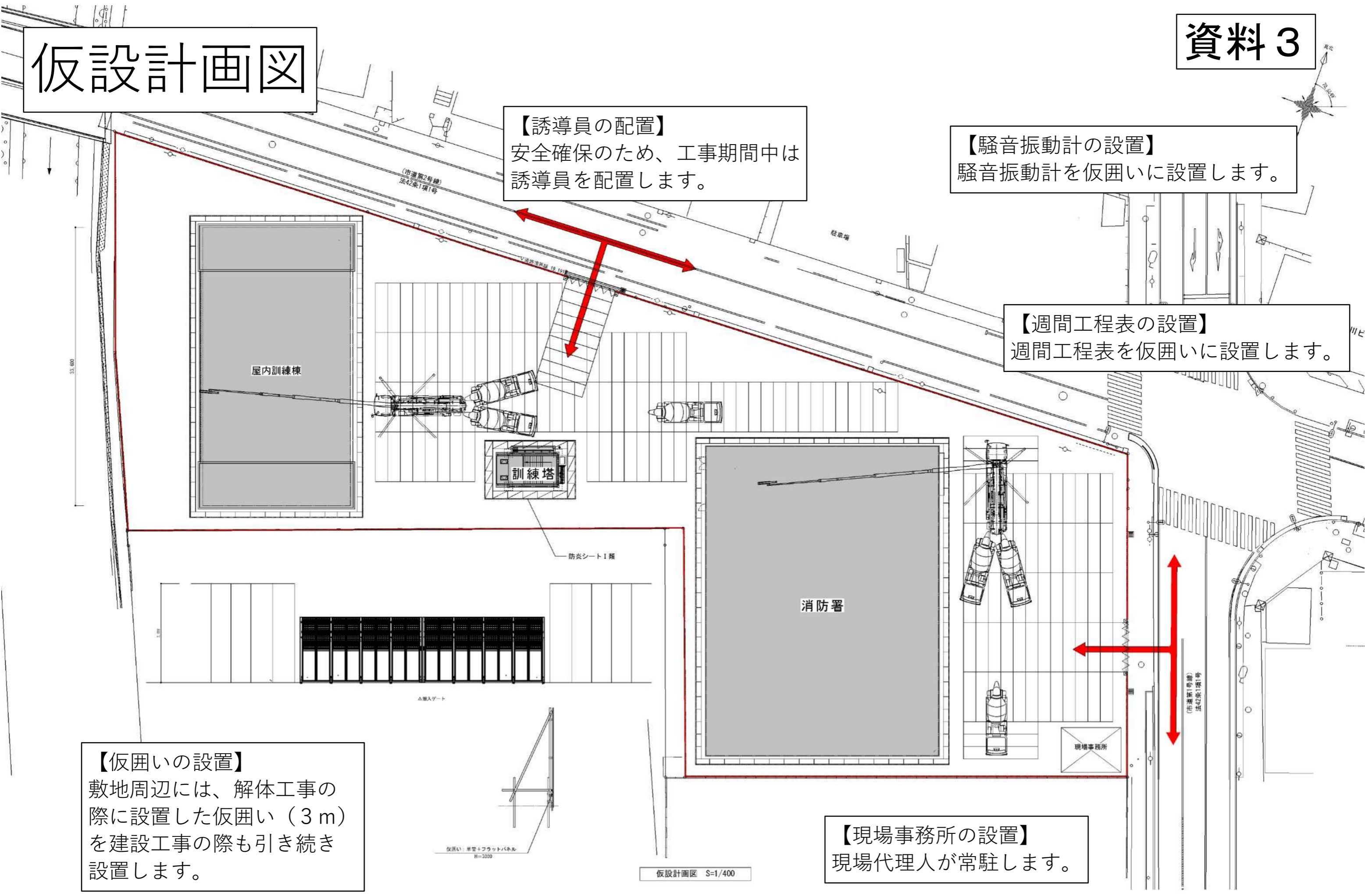
仮設計画図 2
